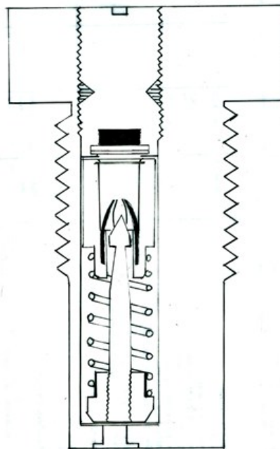
Fusée de 30 mm système Henriët, premiers essais de 1874
