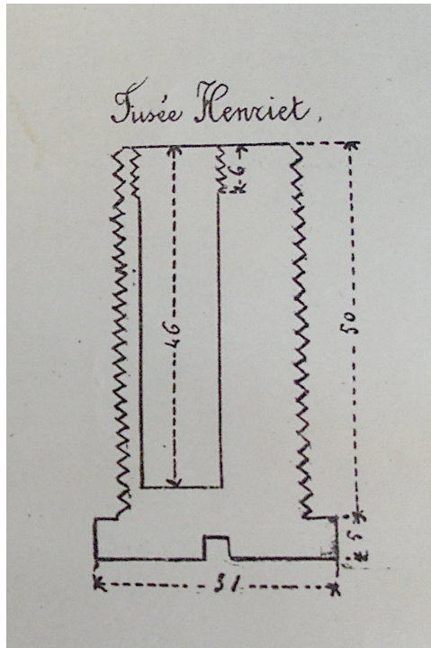
Le percuteur de la fusée Henriet de culot
