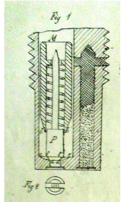
Dessin joint au rapport de la commission de Tarbes — Archives CAA
