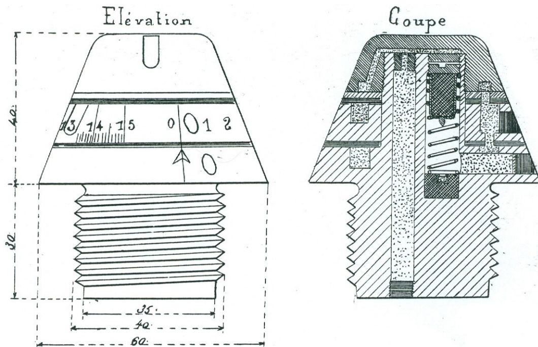
Fusée fusante à cadran et à étage système Henriet de 40mm 1878 — Dessins tirés de Fusées pour projectiles creux -ECP -
