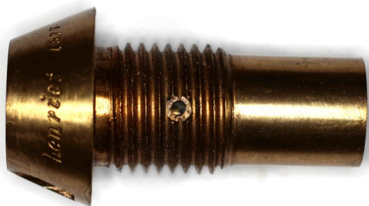
Fusée Henriet N°2 en coupe d'époque à droite , mécanisme au repos. spécimen de coffret à gauche.. On voit sur ce spécimen l'emplacement du trou de perçage établissant la communication entre canal percutant et chambre à poudre allongée.— Photos Philippe Mention© 2020
