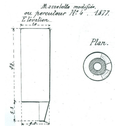
Dessin joint au rapport de la commission de Tarbes — Archives CAA
