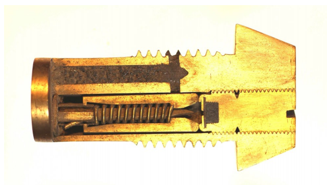
Fusée Henriet N°2 en coupe d'époque à droite , mécanisme au repos. spécimen de coffret à gauche.. On voit sur ce spécimen l'emplacement du trou de perçage établissant la communication entre canal percutant et chambre à poudre allongée.— Photos Philippe Mention© 2020
