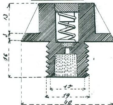
Fusée fusante Henriët pour boîte à mitraille.
