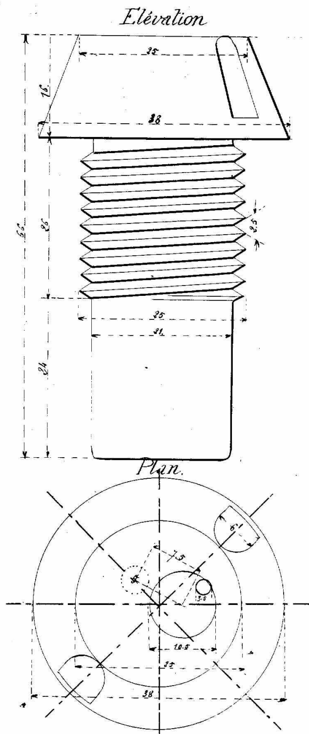
Fusée Henriët à percuteur N° 1 de 1875 modifiée par addition d'une chambre à poudre. - Dessin tiré de Fusées pour projectiles creux 1883 (ECP)
