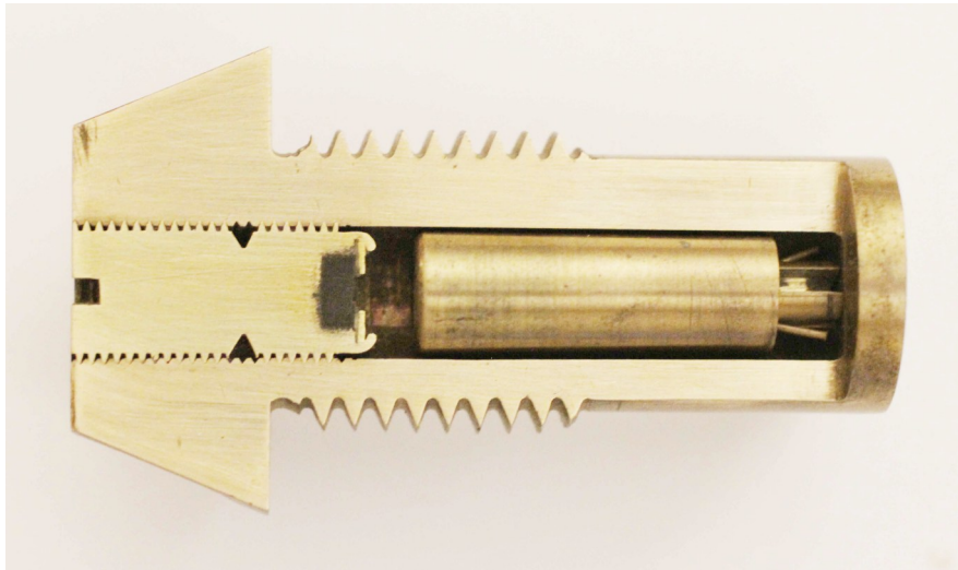
la fusée Henriët de 1874 avec son percuteur modifié. Coupe d'époque. --Photos P. Mention © 2020
